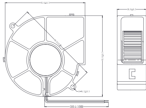
尺寸图 / DIMENSIONS DRAWING
